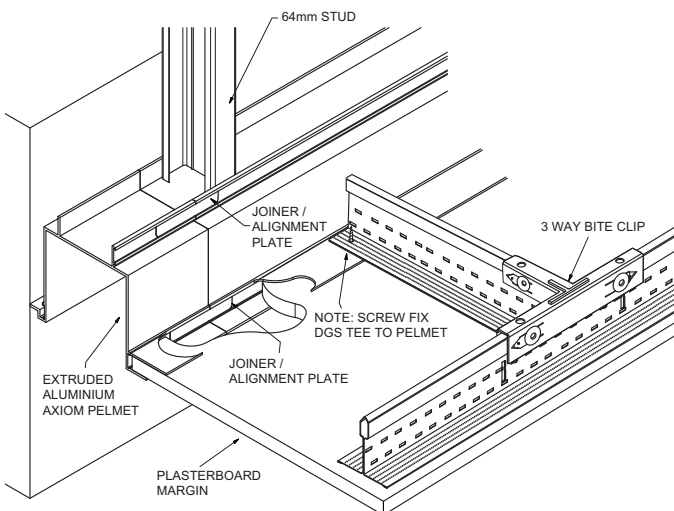
5 Pelmet
