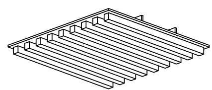
Batten Option 3 - 38 x 28mm
